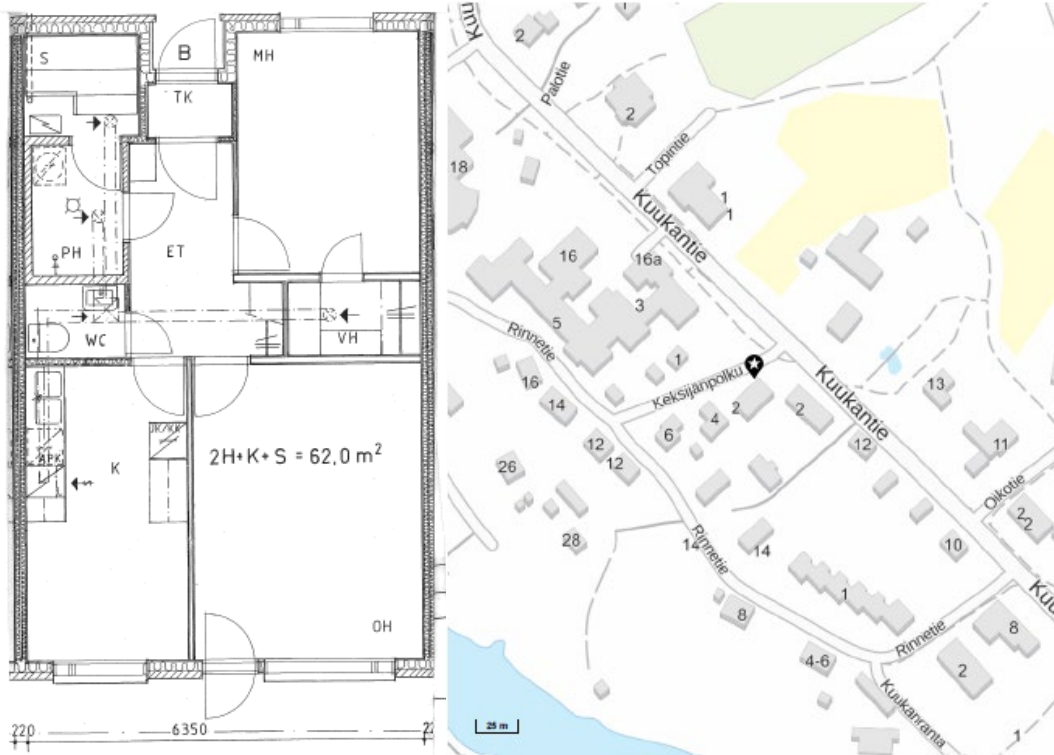
Pohjapiirros
